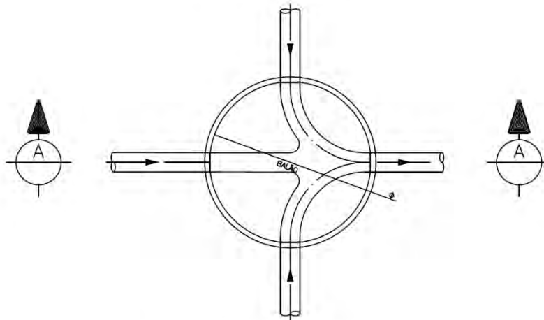
LIGAÇÕES NO FUNDO DO POÇO
