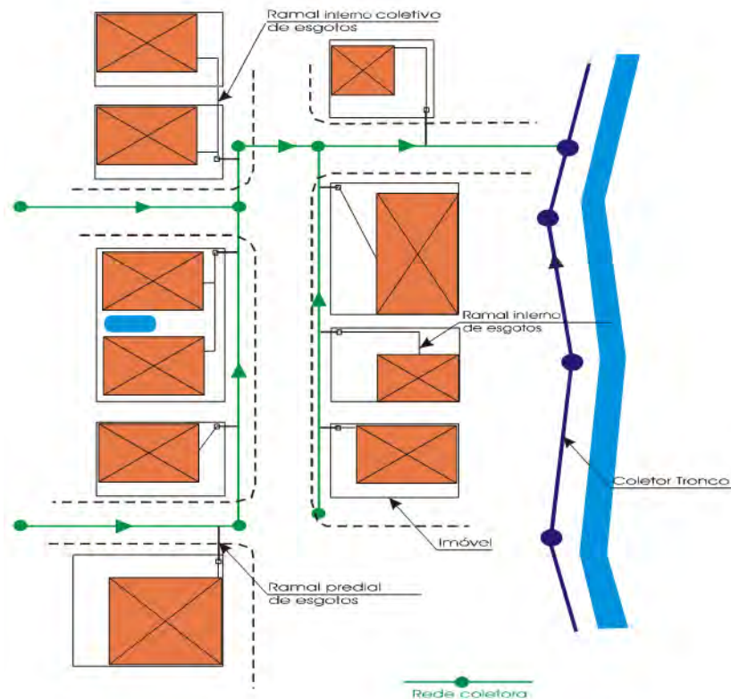
Figura 1 - Desenho esquemático do sistema: ramal, rede coletora e coletor tronco de esgoto.
